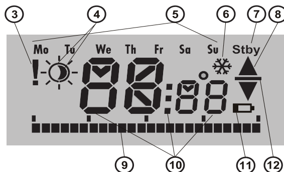
Figure 3: 3 – Entrée de réglages internes depuis F-Link SW/ défaut de communication; 4 – Symboles de température confort Lo et économique Hi ; 5 – Jours de la semaine; 6 – chauffage activé lorsque le thermostat est bloqué; 7 – Mode ARRÊT activé; 8 – Chauffage, clignotement Lo – thermostat bloqué par fenêtre ouverte, par exemple; 9 – Courbe des périodes de chauffage; 10 – Symboles pour afficher la température, l'heure et le texte; 11 – Indicateur de batterie faible; 12 – Affichage de la température pré-réglée / requise
