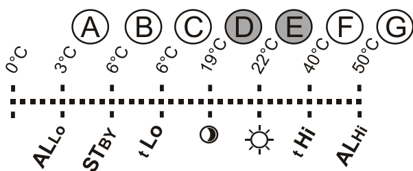
Figure 2: A – Basse température, B – Température en mode ARRÊT, C – Limite de température inférieure pré-réglable par l'utilisateur, D – Température économique, E – Température confort, F – Limite de température supérieure pré-réglable par l'utilisateur, G – Température élevée
